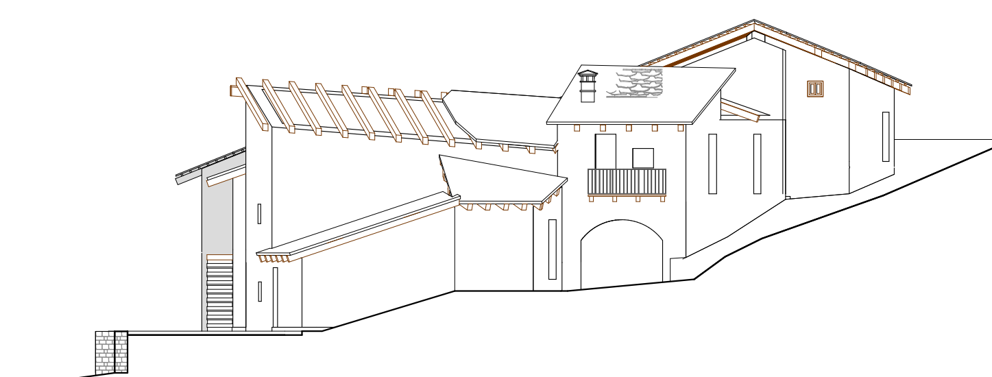
PROSPETTO EST
