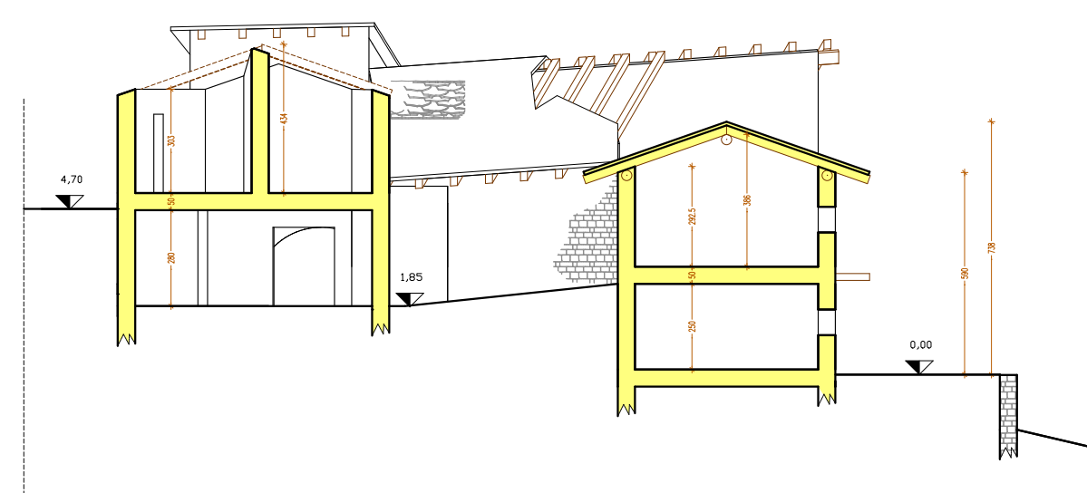
Sezione B-3 ( Post Modifica )
