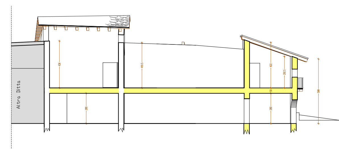
SEZIONE E-E
