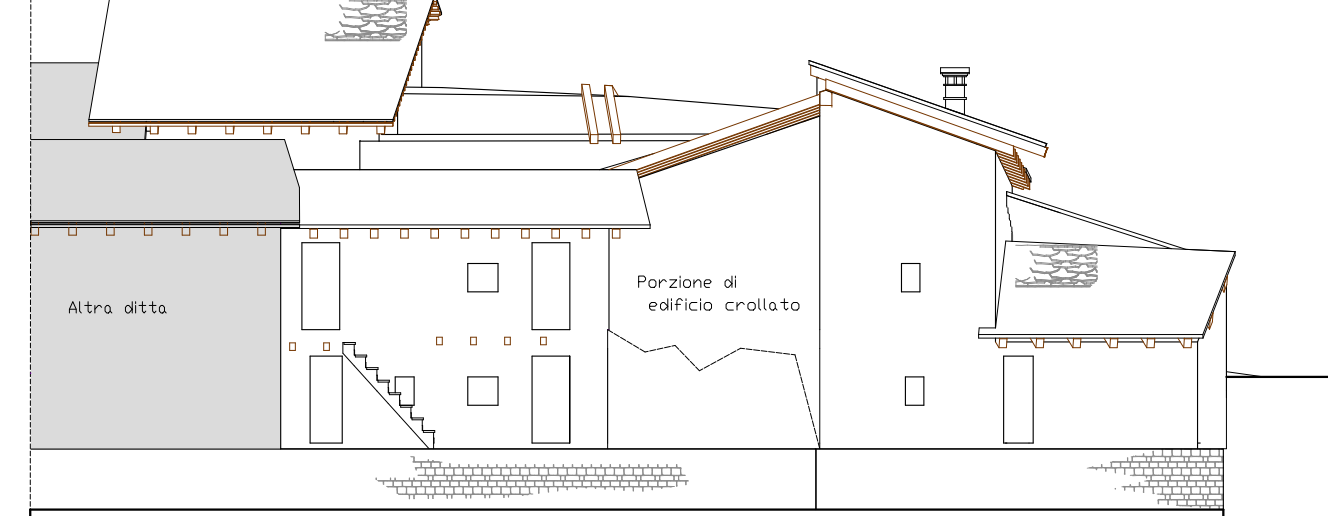
PROSPETTO SUI < Ante Modifica >
