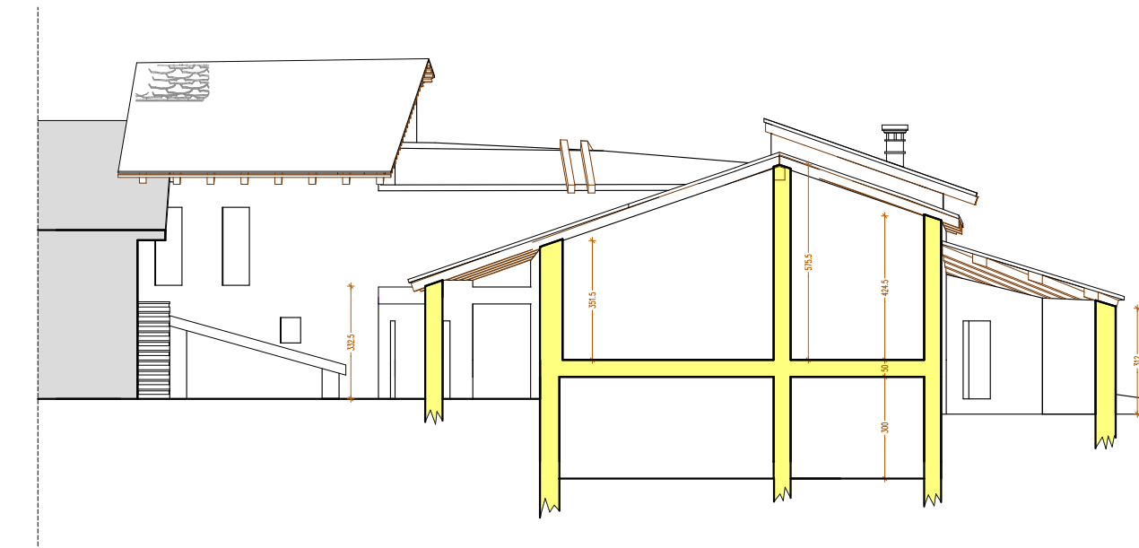
SEZIONE D- < Post Modifica >
